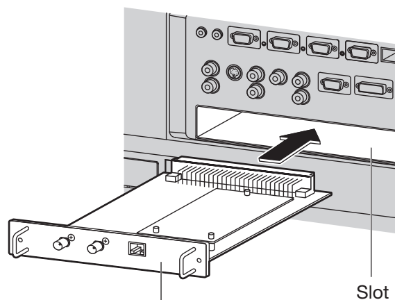
Input module
