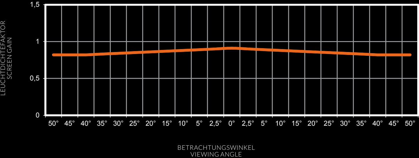
LEUCHTDICHTEFAKTOR NACH DIN 19045 | GAIN ACCORDING TO DIN 19045 STRATO ECO JMB
