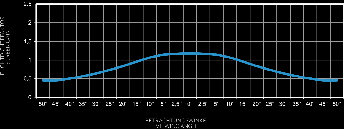
LEUCHTDICHTEFAKTOR NACH DIN 19045 | GAIN ACCORDING TO DIN 19045 FLEX REAR-CI
