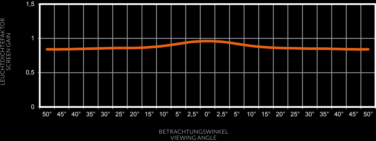
LEUCHTDICHTEFAKTOR NACH DIN 19045 | GAIN ACCORDING TO DIN 19045 STRATO TK
