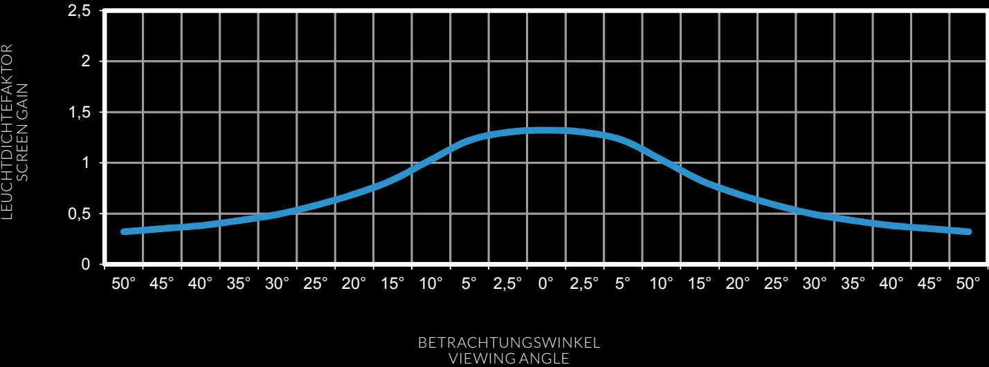
LEUCHTDICHTEFAKTOR NACH DIN 19045 | GAIN ACCORDING TO DIN 19045 FLEX REAR CIX
