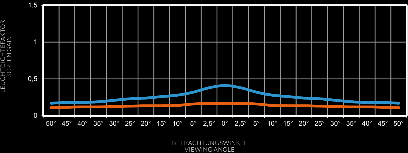
LEUCHTDICHTEFAKTOR NACH DIN 19045 | GAIN ACCORDING TO DIN 19045 FLEX DUAL BLACK
