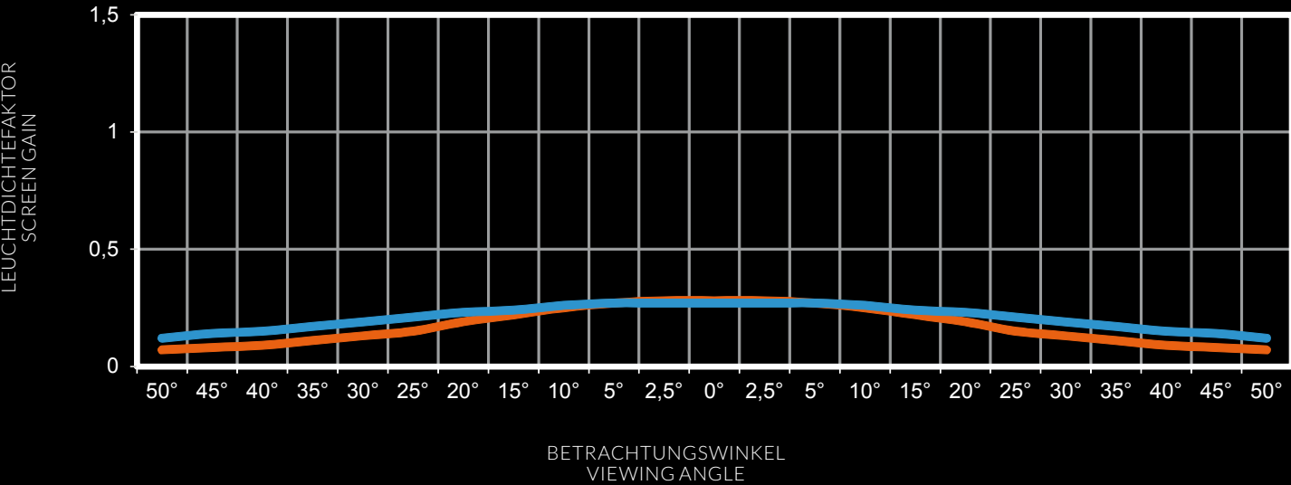
LEUCHTDICHTEFAKTOR NACH DIN 19045 | GAIN ACCORDING TO DIN 19045 FLEX DUAL BLACK PRO
