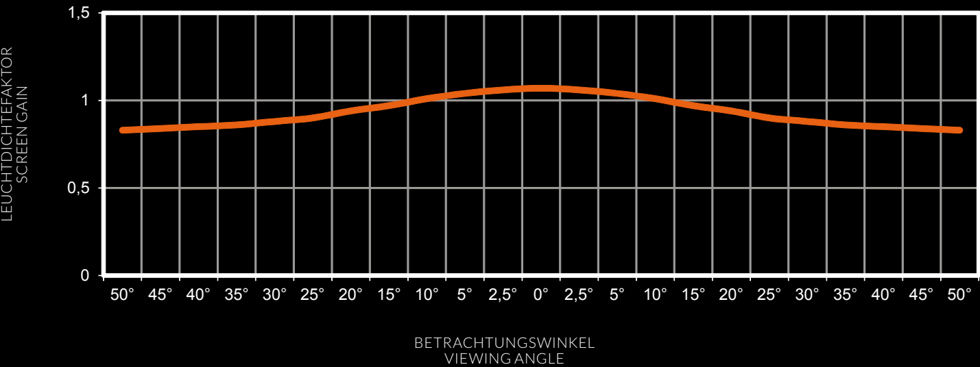
LEUCHTDICHTEFAKTOR NACH DIN 19045 | GAIN ACCORDING TO DIN 19045 FLEX WHITE MO
