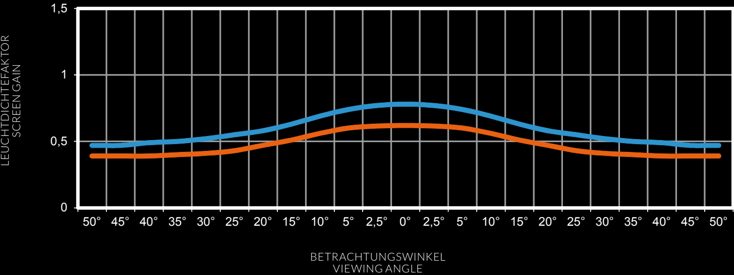
LEUCHTDICHTEFAKTOR NACH DIN 19045 | GAIN ACCORDING TO DIN 19045 FLEX DUAL MO multi image
