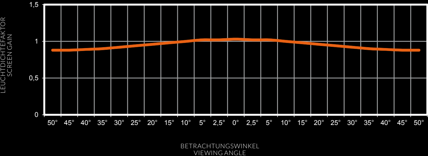
LEUCHTDICHTEFAKTOR NACH DIN 19045 | GAIN ACCORDING TO DIN 19045 FLEX WHITE CI
