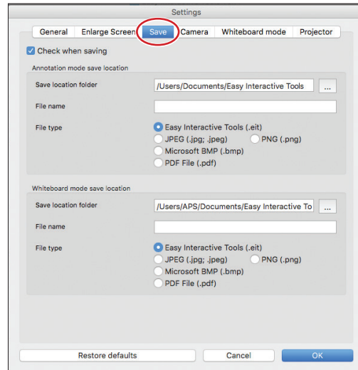
OS X
